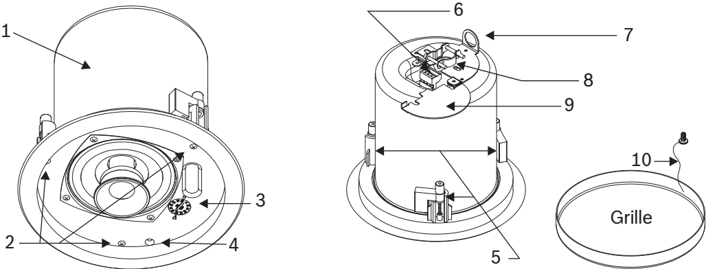
Abbildung 3.2: Unterseite des Lautsprechers (links); Oberseite des Lautsprechers (Mitte); Gitter (rechts)
