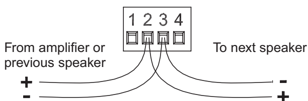
Abbildung 4.6: Parallele Verdrahtung
