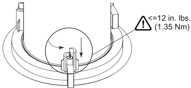
Abbildung 4.14: Befestigungslaschen festziehen
