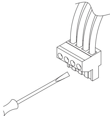
Abbildung 4.5: Mit Schraubendreher festziehen
