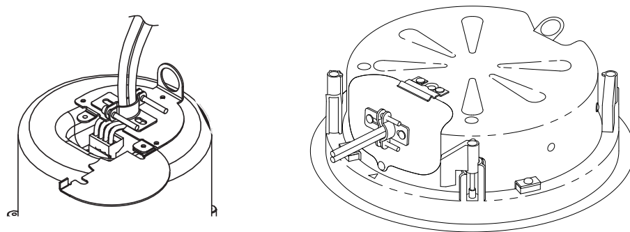
Abbildung 4.11: Befestigen Sie das Kabel durch die Versraubung außer C4.2LP (links); befestigen Sie das Kabel durch die Versraubung für den C4.2LP (rechts)
