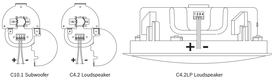
Abbildung 4.8: Subwoofer-Polarität mit C4.2/C4.2LP
