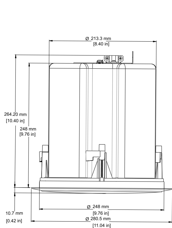
EVID PC6.2 - Dimensioni
