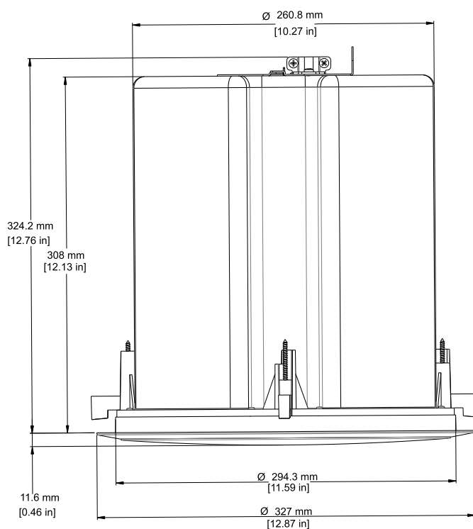
EVID PC8.2 - Dimensioni
