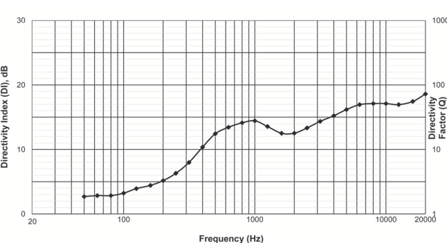
EVID PC6.2 - Direzionalità
