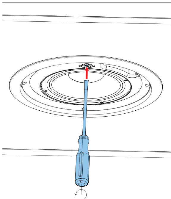
Figura 4.11: regolare il selettore
