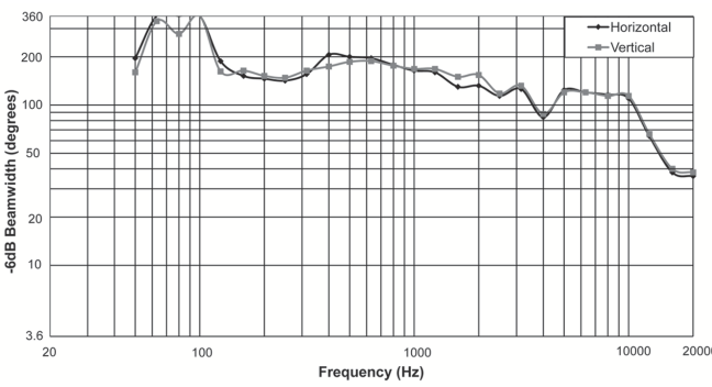
EVID PC8.2 - Ampiezza raggio
