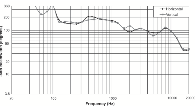
EVID PC6.2 - Ampiezza raggio
