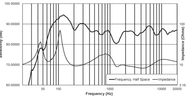
EVID PC6.2 - Risposta in frequenza e impedenza
