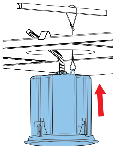
Figura 4.8: installare gli altoparlanti nel soffitto
