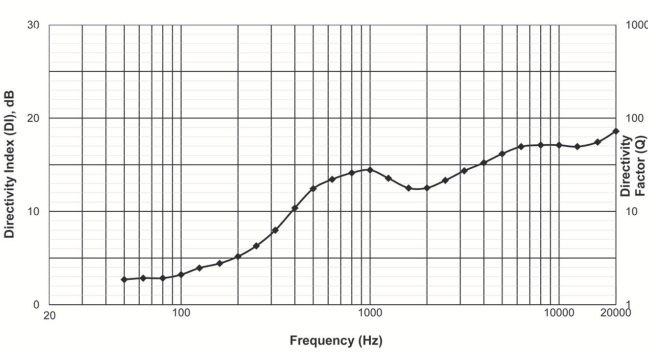
EVID PC8.2 - Direzionalità
