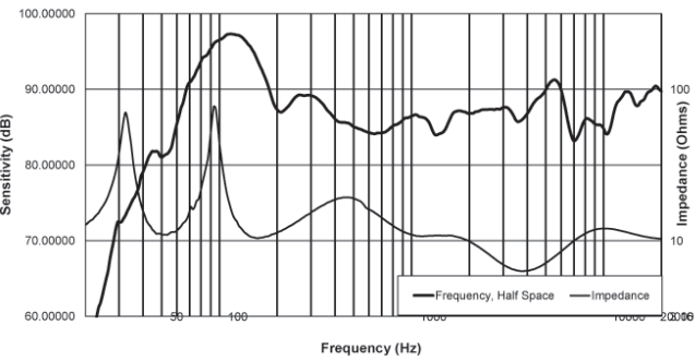
EVID PC8.2 - Risposta in frequenza e impedenza
