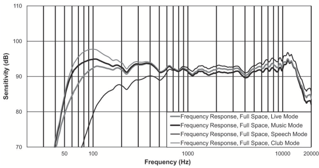
频率响应:
