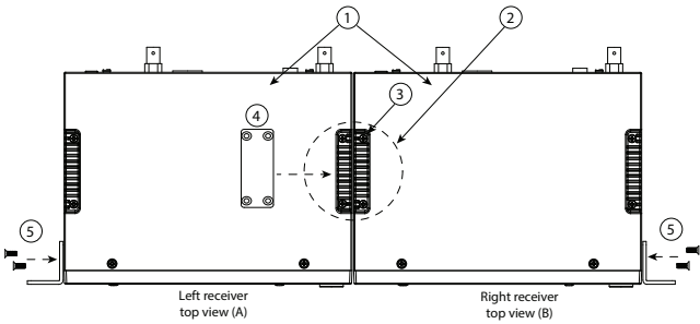
A 左接收器俯视图 B 右接收器俯视图
