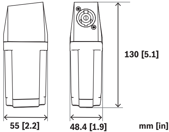
Fig. 3: Adaptateur pour caisson de basse pour EVOLVE-WMK avec connecteur NL4
