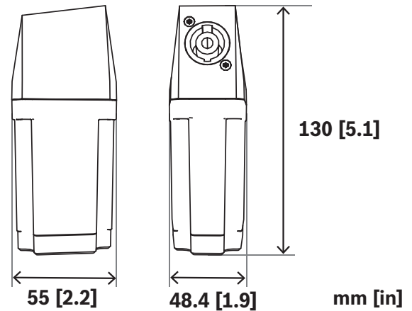
図. 3: EVOLVE-WMK 用サブウーファアダプター、NL4 コネクタ付き
