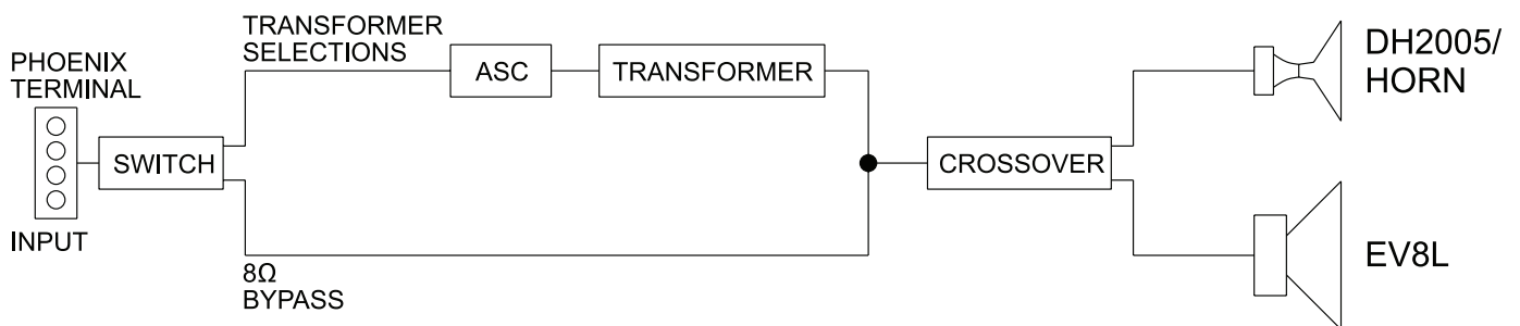
Abb. 2: ZX1i (mit Transformator)
